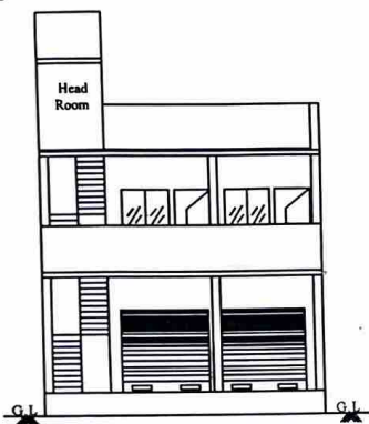
ELEVATION
