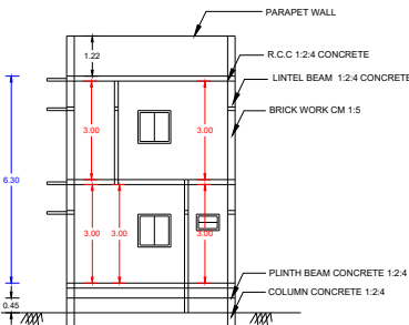
SECTION A-B
