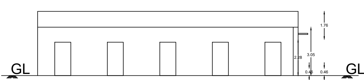
ELEVATION - A
