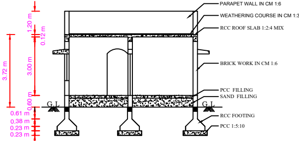
SECTION - AB
