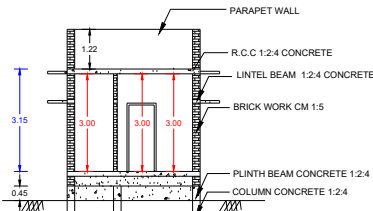
SECTION A-B
