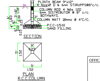
R.C.C.COLUMN
