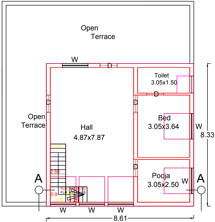
PLAN - F.F
