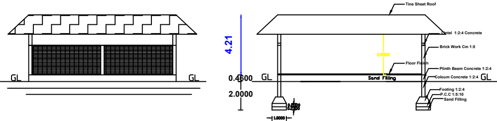
Elevation
