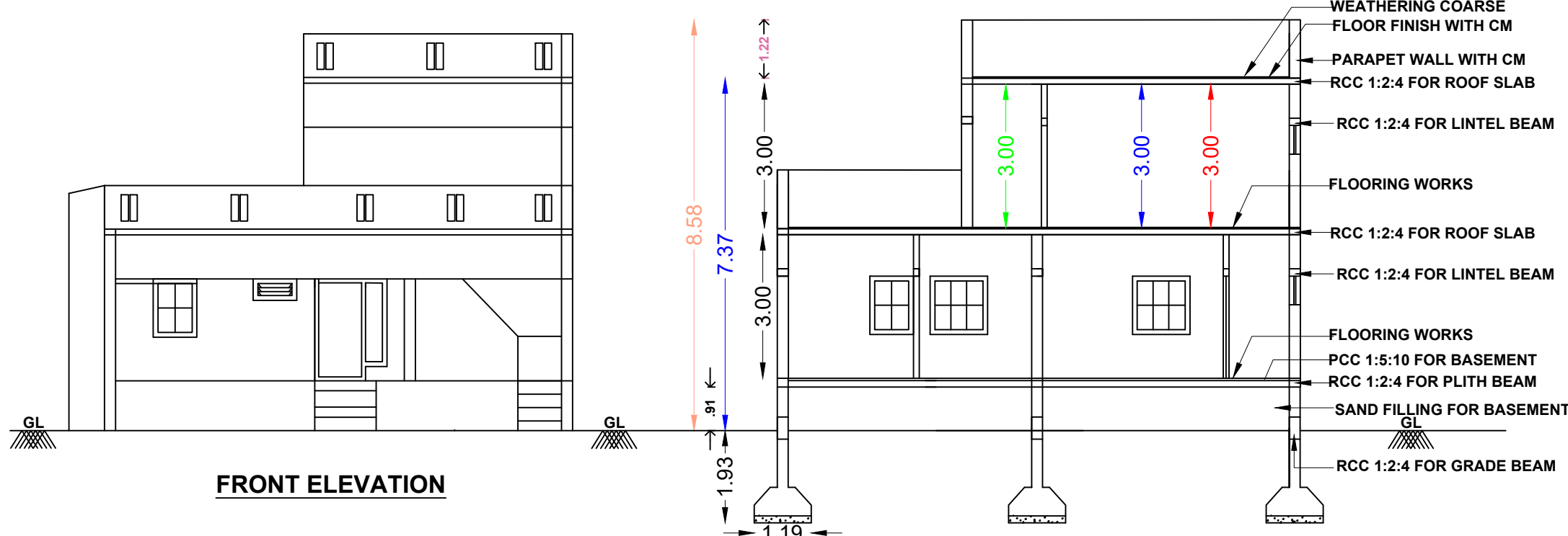
SECTION A-A
