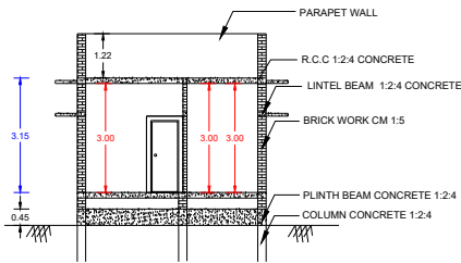
SECTION A-B
