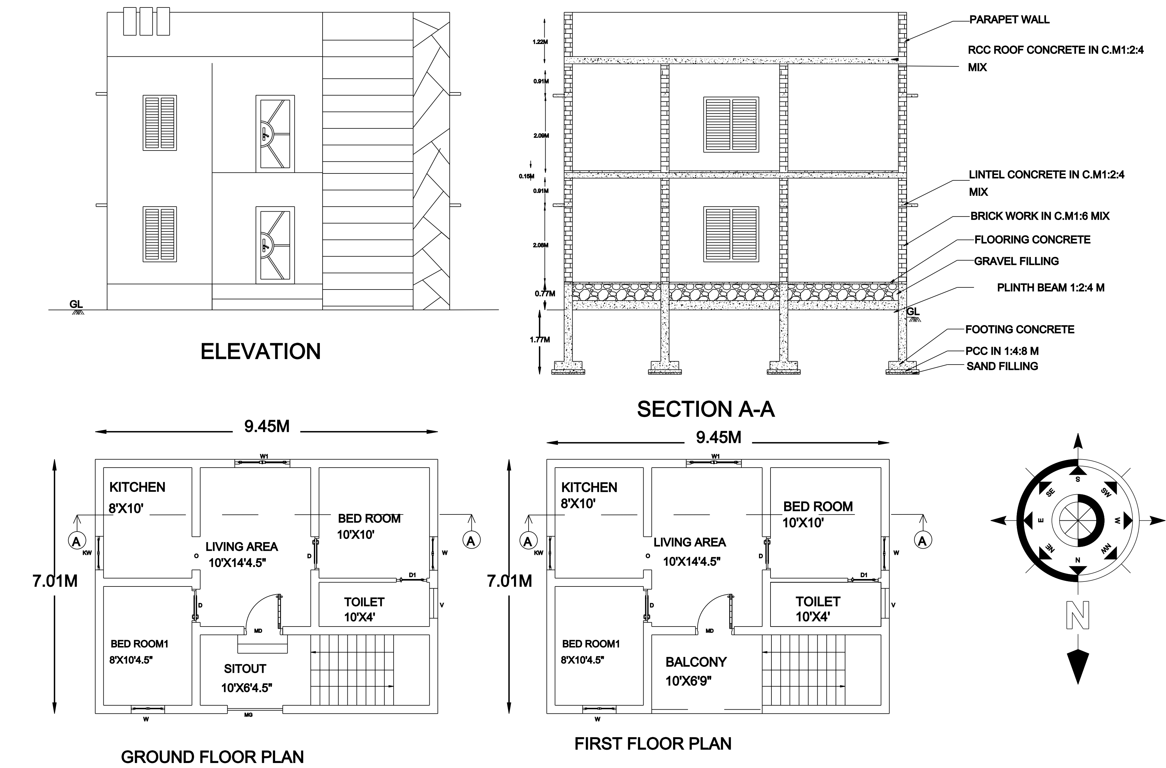
SCALE - 1 : 100
