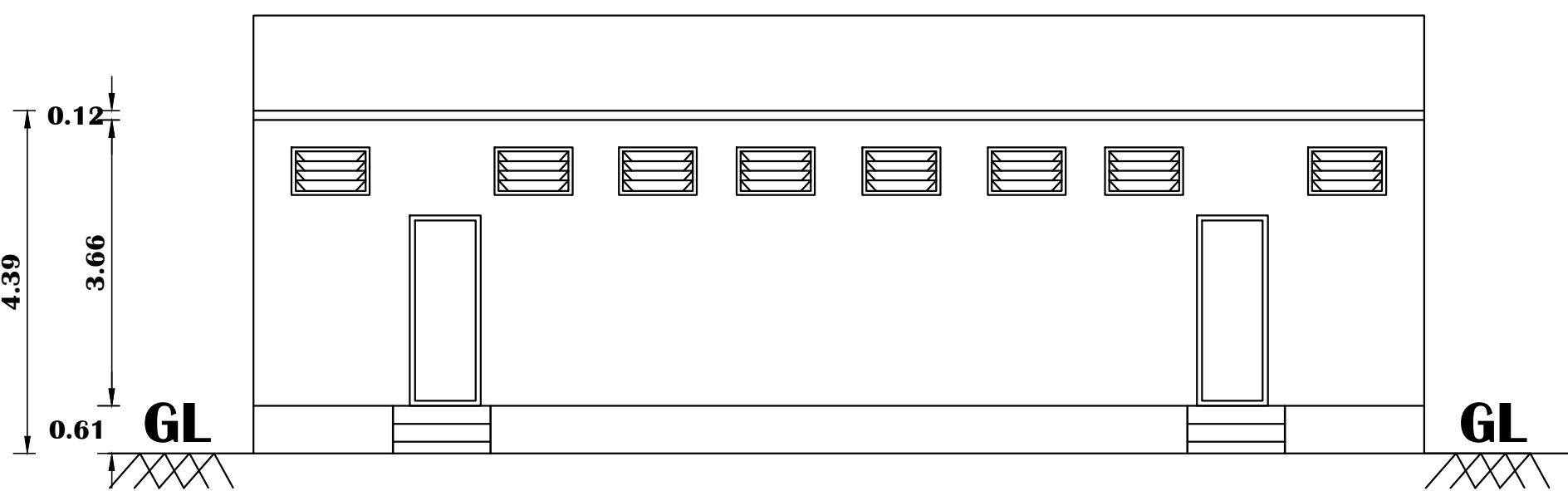
ELEVATION
