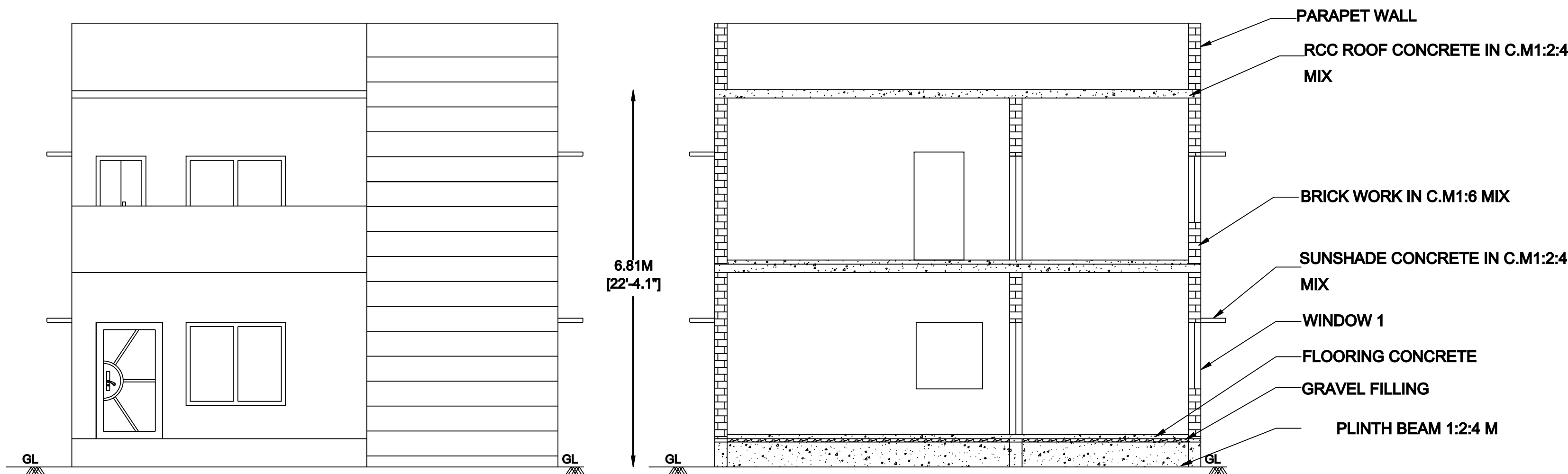
ELEVATION
