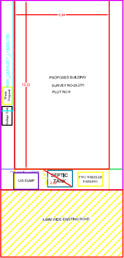
SITEPLAN
