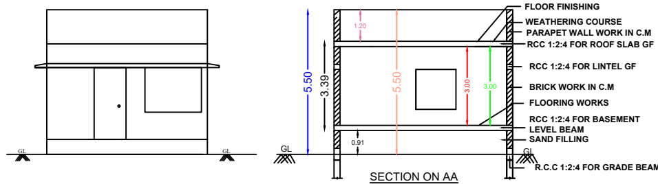
ELEVATION
