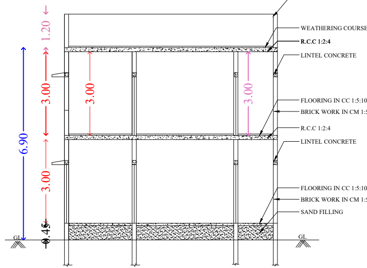
SECTION A-B
