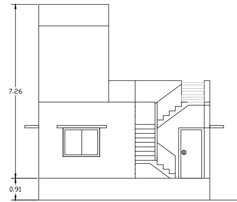
ELEVATION -1
