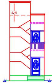
ELEVATION
