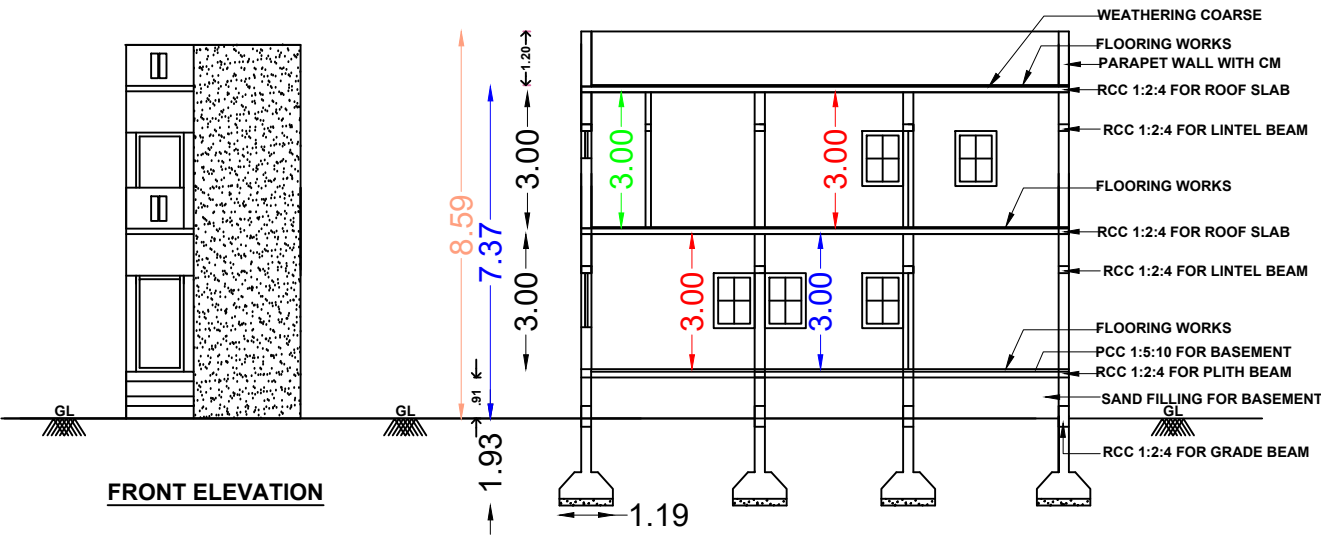
SECTION A-A
