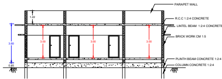
SECTION A-B
