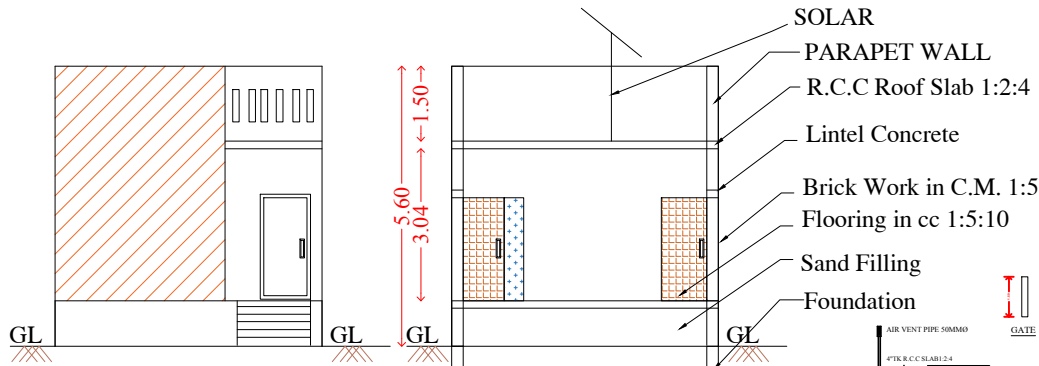
Elevation
