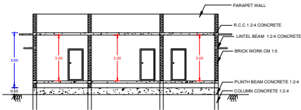
SECTION A-B
