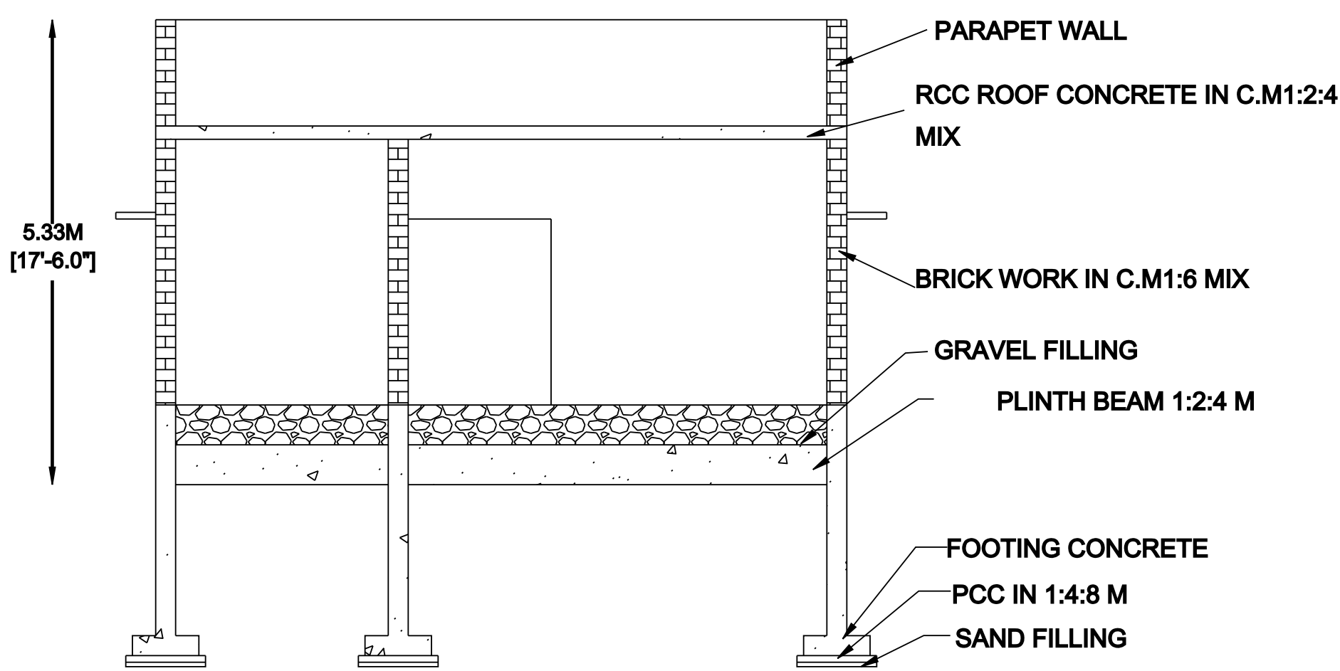
SECTION A-A
