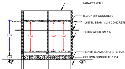
SECTION A-B
