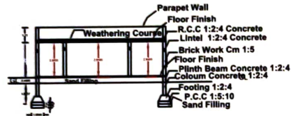
SECTION - AB
