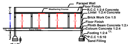
SECTION - AB
