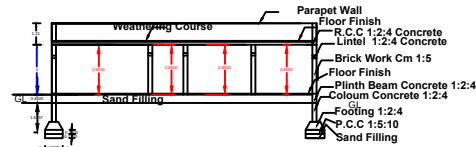
SECTION - AB
