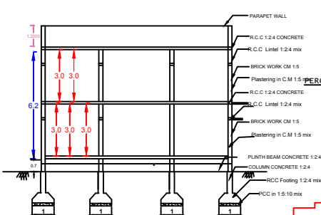
SECTION A-B
