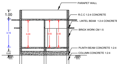
SECTION A-B
