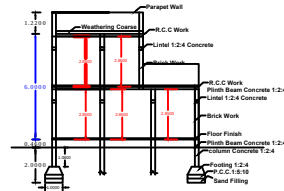
SECTION - AB
