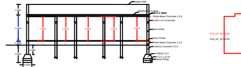
SECTION - AB
