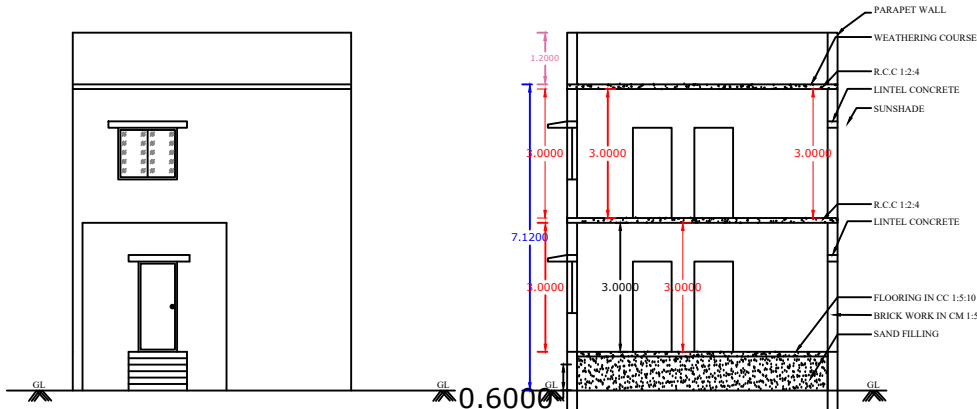
ELEVATION
