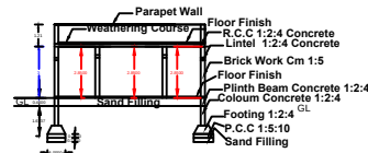
SECTION - AB
