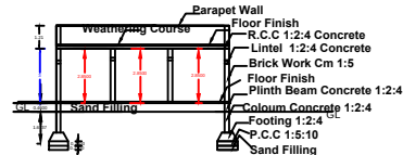
SECTION - AB
