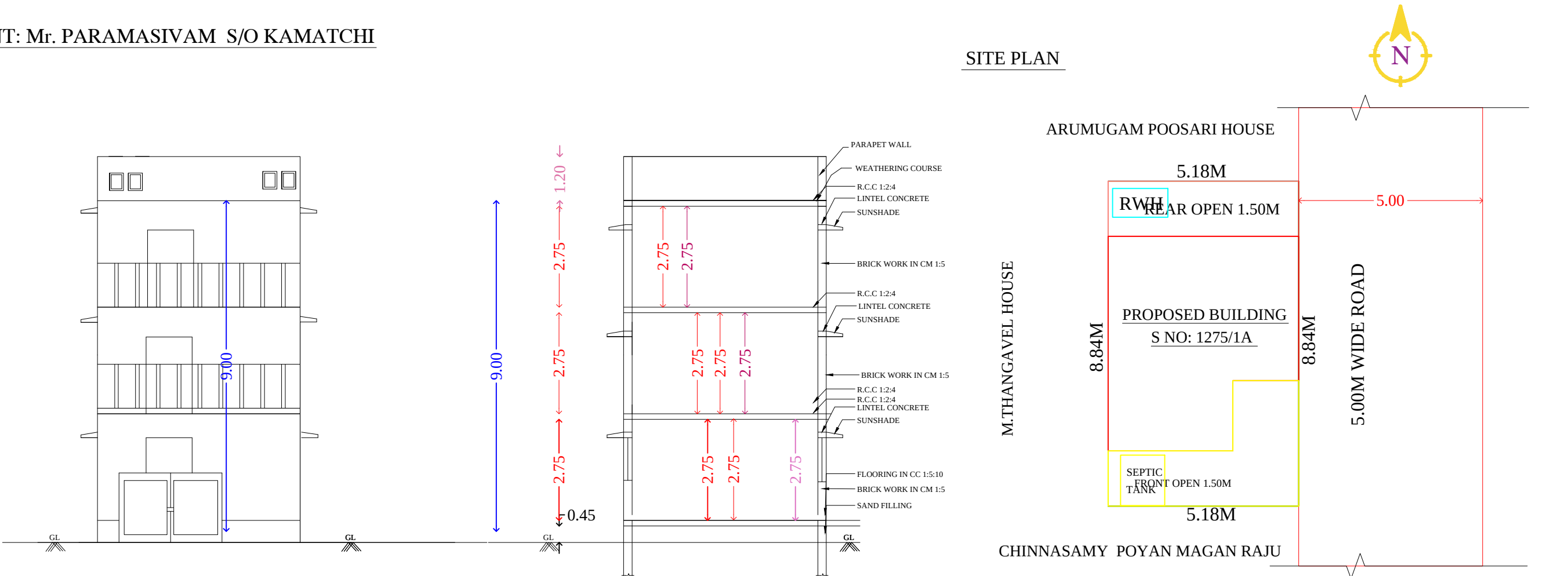
ELEVATION
