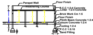
SECTION - AB
