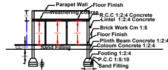
SECTION - AB
