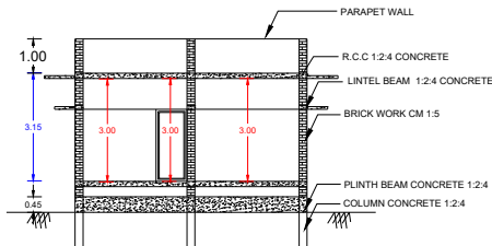
SECTION A-B
