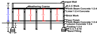
SECTION - AB
