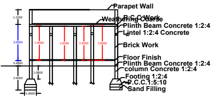
SECTION - AB
