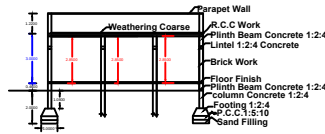
SECTION - AB
