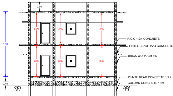
SECTION A-B
