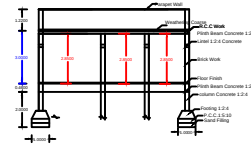
SECTION - AB
