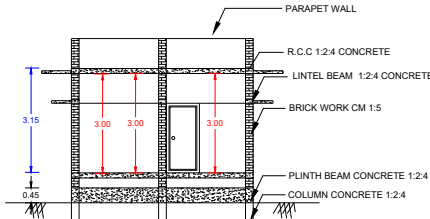
SECTION A-B
