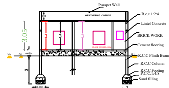
SECTION - AB
