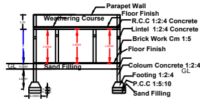
SECTION - AB
