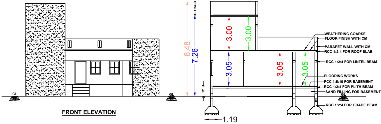
SECTION A-A
