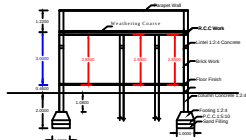
SECTION - AB
