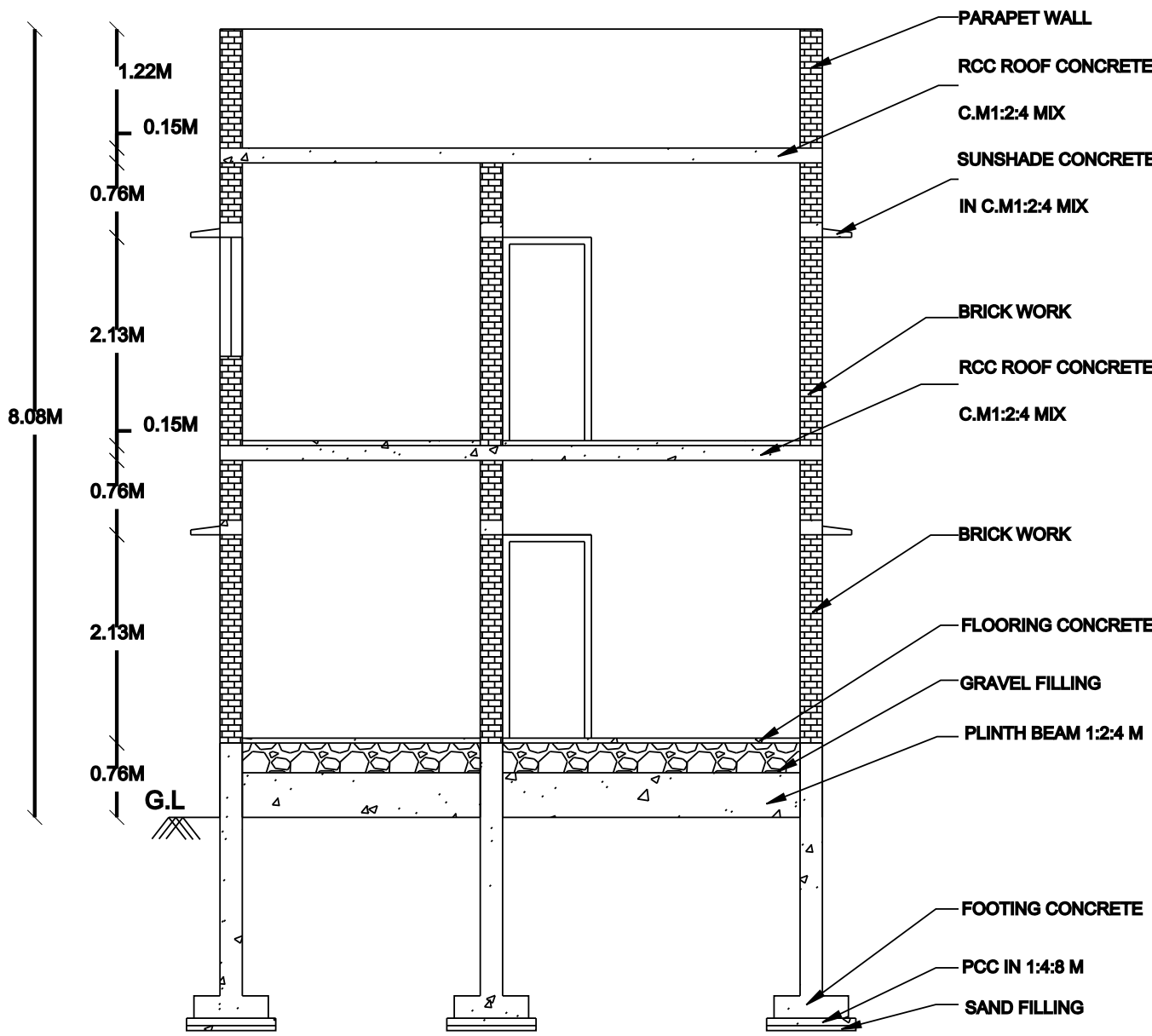
SECTION A-B
