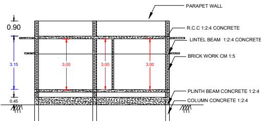
SECTION A-B
